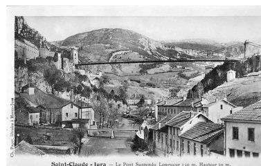
Saint-Claude - Jura - Le Pont suspendu. Longueur 150 m. Hauteur 50 m. Phot. Jérôme Mongreville IVR43_19913900075X
