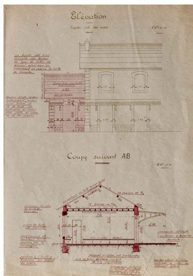
Gare de Lavans - St Lupicin. Amélioration des installations GV et PV [détail : coupe et élévation], 1926. Phot. Yves Sancey, Autr. P. (ingénieur civil) NEPASUTILISEROudotte IVR43_20073900364NUCA
