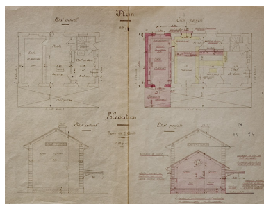
Gare de Lavans - St Lupicin. Amélioration des installations GV et PV [détail : plans et élévations], 1926. Phot. Yves Sancey, Autr. P. (ingénieur civil) NEPASUTILISEROudotte IVR43_20073900365NUCA
