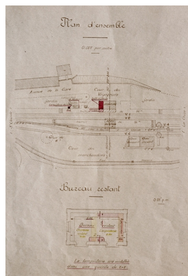
Gare de Lavans - St Lupicin. Amélioration des installations GV et PV [détail : plans], 1926. Phot. Yves Sancey, Autr. P. (ingénieur civil) NEPASUTILISEROudotte IVR43_20073900363NUCA
