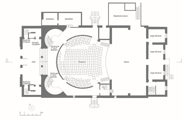
Plan au rez-de-chaussée. D'après un plan de Jérôme Sabre. Dess. Aline Thomas, Autr. Jérôme Sabre IVR26_20222100158NUDA
