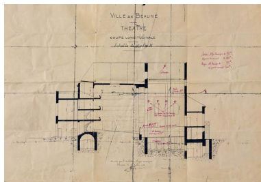
Ville de Beaune. Théâtre. Coupe longitudinale [plan surchargé à l'encre rouge d'indications se rapportant à l'éclairage de la cage de scène]. 24 juillet 1933. Phot. Pierre-Marie Barbe- Richaud, Autr. Abel Lobot IVR26_20222100374NUC4A
