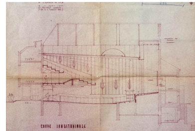
Cinéma Rex à Beaune. 800 places. Avant projet. [Détail :] Coupe longitudinale. 1er avril 1951. Autr. Georges Peynet, Phot. Pierre-Marie Barbe-Richaud IVR26_20222100381NUC4A
