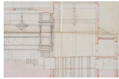
Ville de Beaune. Projet de théâtre. Coupe longitudinale [détail : la scène]. 1er mars 1860. Phot. Pierre-Marie Barbe- Richaud, Autr. Félix Goin IVR26_20222100373NUC4A
