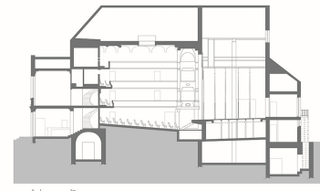
Coupe longitudinale. D'après une coupe de Jérôme Sabre. Dess. Aline Thomas, Autr. Jérôme Sabre IVR26_20222100159NUDA
