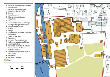
Plan-masse de l'usine vers 1998. Dess. Mathias Papigny IVR43_20142500613NUDA
