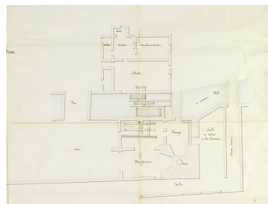
Plan géométrique du moulin de Saint-Loup-lès-Gray, des bâtiments qui en dépendent [...] appartenant à M. le Baron de Klinglin. Phot. Jérôme Mongreville IVR43_20097000033NUC2A
