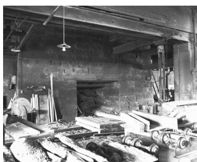
Mur nord du haut fourneau (ouverture de la tuyère) en 1990. Phot. Yves Sancey IVR43_19907000111X
