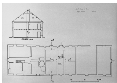
Plan et coupe du rez-de-chaussée du logement ouvrier. Relevé graphique, 1993, M. Brugier et F. Corbineau, échelle 1:1250. Phot. Jérôme Mongreville IVR43_19937000009X
