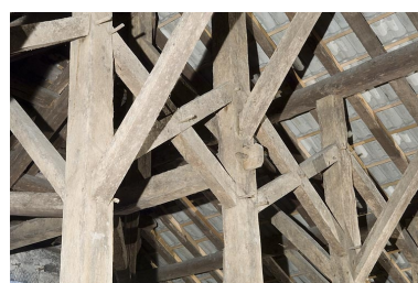
Charpente du fenil. Détail de partie haute (contrefiches et croix de Saint-André). Phot. Jérôme Mongreville IVR43_20067000790NUCA
