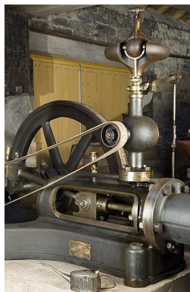
Machine à vapeur Diebold et Michel (Nancy). Détail. Phot. Jérôme Mongreville IVR43_20067000807NUCA
