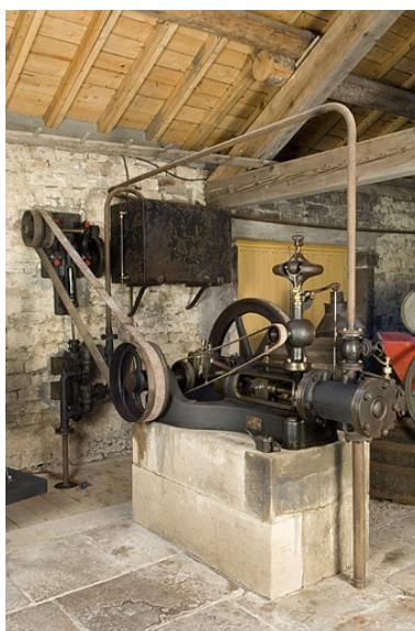
Machine à vapeur Diebold et Michel (Nancy). Vue d'ensemble. Phot. Jérôme Mongreville IVR43_20067000806NUCA
