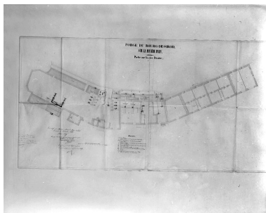
Forge du Bourg de Sirod, sur la rivière d'Ain. Partie sur la rive Droite. Phot. Yves Sancey IVR43_19973901996V
