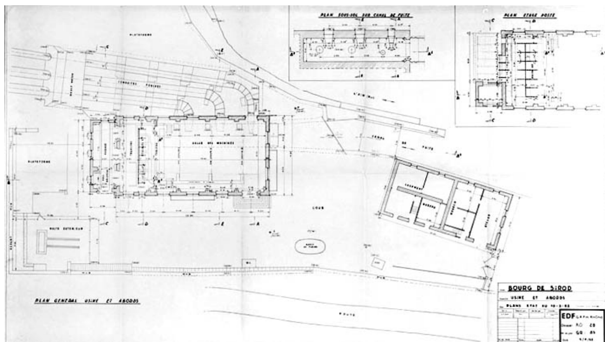
Usine et abords. Plans. Etat au 10-3-62.
