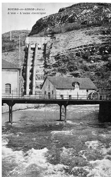
Bourg-de-Sirod (Jura). L'Ain - L'usine électrique. Phot. Jérôme Mongreville, Phot. G. Karrer IVR43_19913900197X
