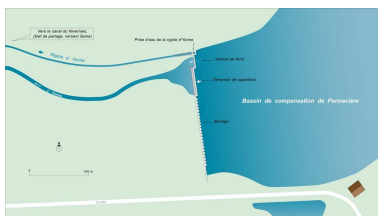
Carte schématique du bassin de compensation et de la prise d'eau de la rigole d'Yonne. Dess. Alain Morelière IVR26_20145800014NUDA
