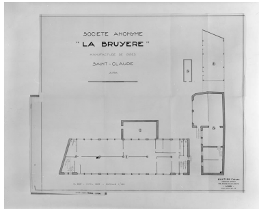
Société Anonyme "La Bruyère", manufacture de pipes. Saint Claude. Jura [plan de distribution au rez-de-chaussée]. Phot. Jérôme Mongreville, Autr. Galtier Frères et Cie IVR43_19923900012V
