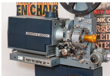
Lanterne et bloc de projection. Phot. Pierre-Marie Barbe-Richaud IVR26_20245800321NUC4A
