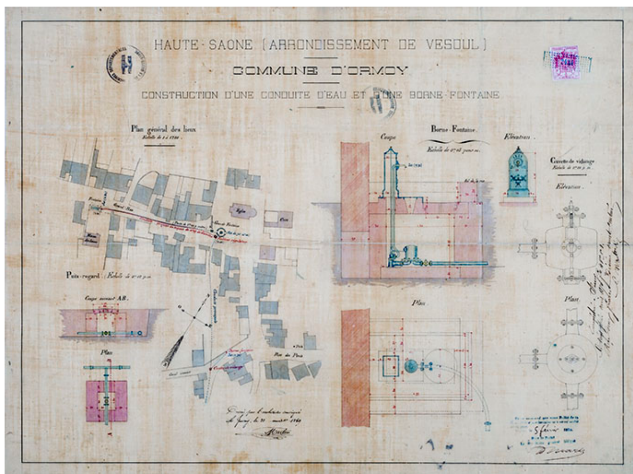
Construction d'une borne-fontaine et d'une conduite d'eau (1869).
