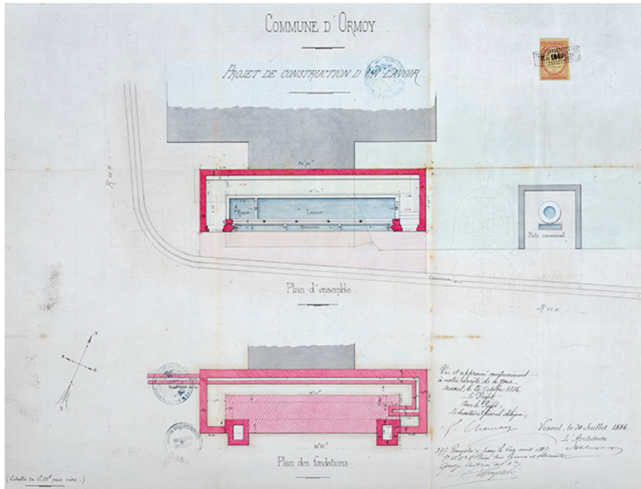
Projet de construction d'un lavoir (1886).
