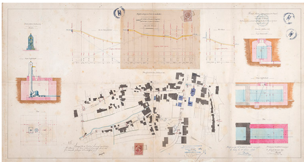
Projet de construction de bornes-fontaines (1891).
