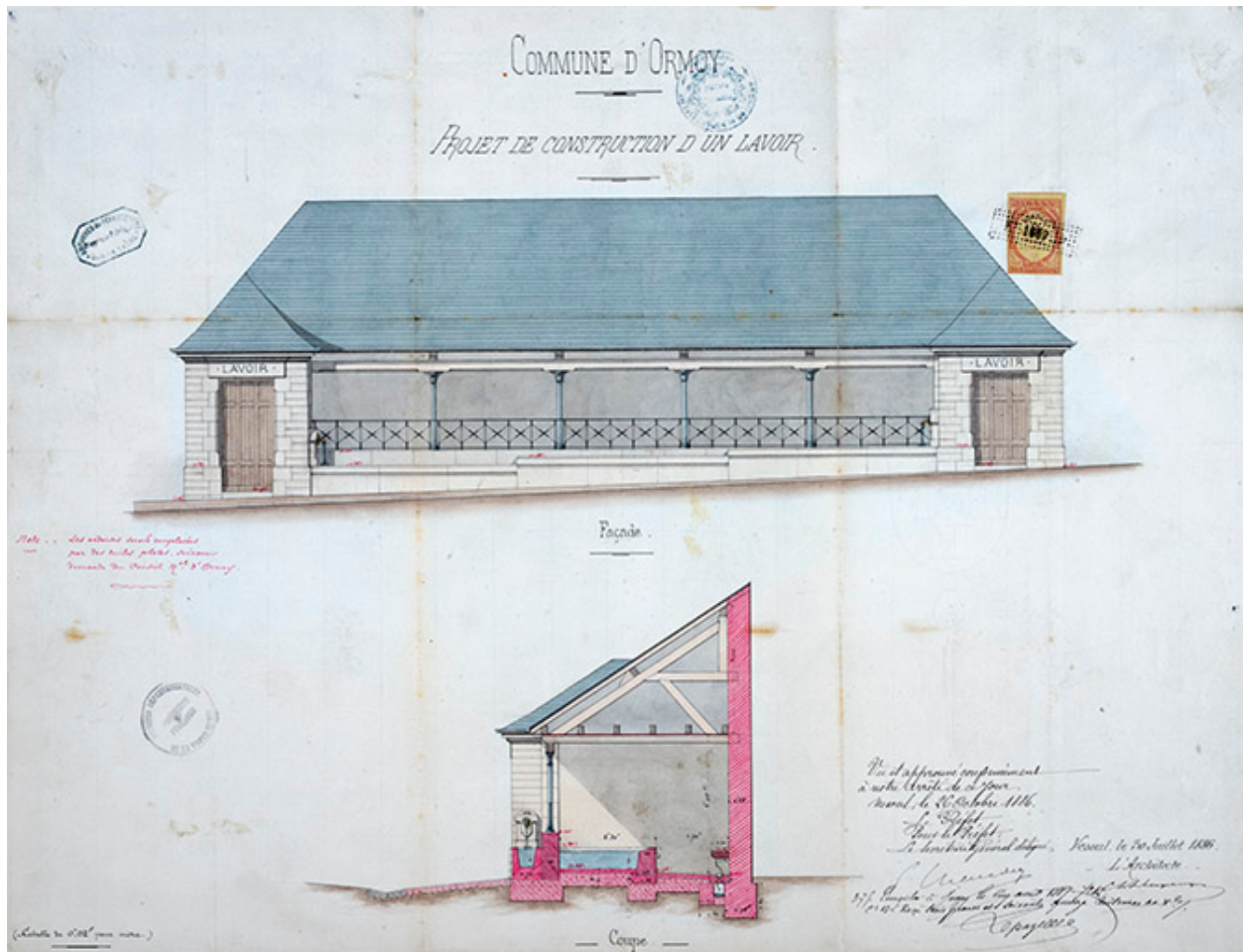
Projet pour le lavoir rue des Vignes (1886).
