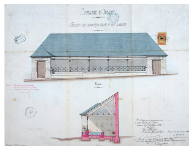
Projet pour le lavoir rue des Vignes (1886). Phot. Jérôme Mongreville, Autr. Charles Desgranges IVR43_20167000959NUC4A
