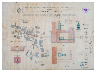
Construction d'une borne-fontaine et d'une conduite d'eau (1869). Phot. Jérôme Mongreville, Autr. J.-B. Martin
