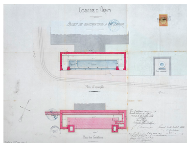
Projet de construction d'un lavoir (1886). Phot. Jérôme Mongreville, Autr. Charles Desgranges IVR43_20167000957NUC4A
