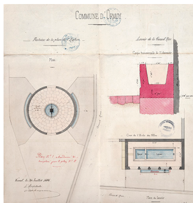
Plans proposés pour l'édification d'une fontaine au centre du village et d'un abreuvoir, Grande rue (1886). Phot. Jérôme Mongreville, Autr. Charles Desgranges IVR43_20167000958NUC4A
