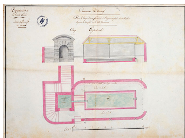
Projet de construction de la fontaine-lavoir en bord de Saône (1821). Phot. Jérôme Mongreville, Autr. Ponsard
