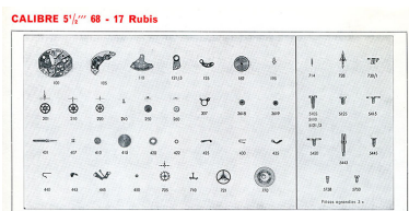
Calibre 5 1/2''' 68 - 17 rubis [éclaté des fournitures], 1973.
