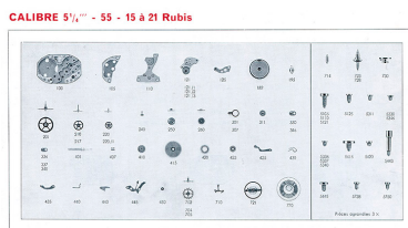
Calibre 5 1/4''' - 55 - 15 à 21 rubis [éclaté des fournitures], 1973. Autr. auteur inconnu IVR43_20162500141NUC2A
