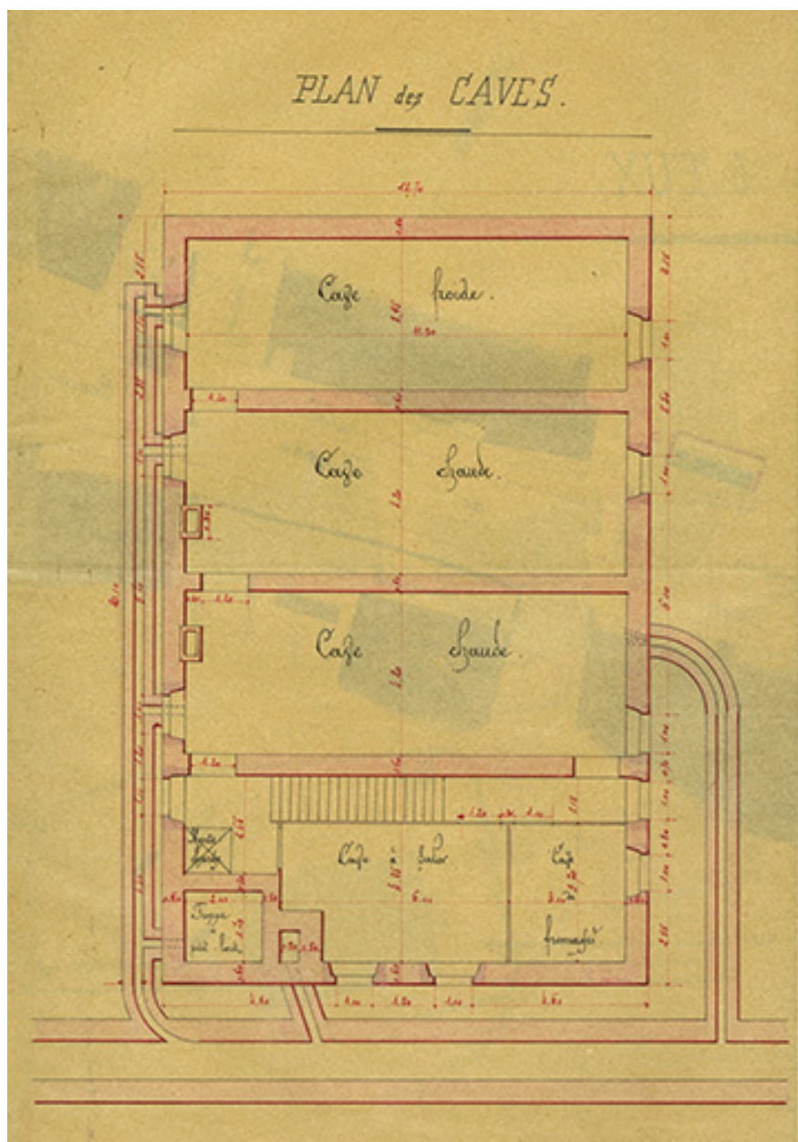
Construction d'un chalet-modèle. Plan des caves, 1901.
