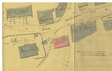
Construction d'un chalet-modèle. Plan de situation, 1901 IVR43_20192500099NUC4A
