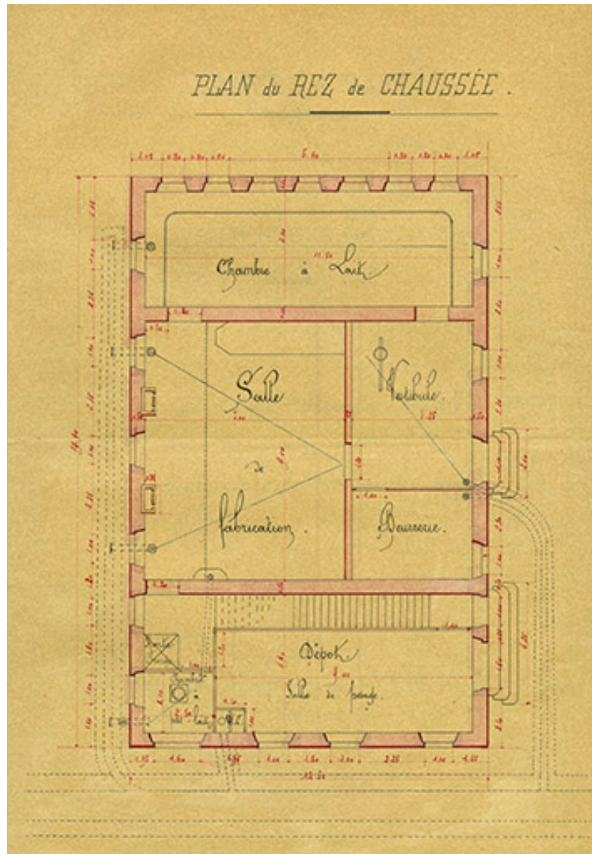
Construction d'un chalet-modèle. Plan du rez-de-chaussée, 1901.
