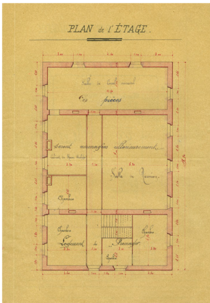
Construction d'un chalet-modèle. Plan de l'étage, 1901.
