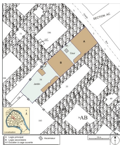
Plan masse et de situation. Extrait du plan cadastral, 1974, section AB. Dess. André Céréza IVR43_20072500100NUDA
