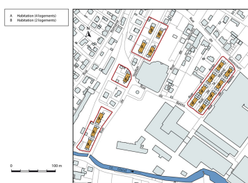
Plan-masse et de situation. Dess. Mathias Papigny IVR43_20132502540NUDA
