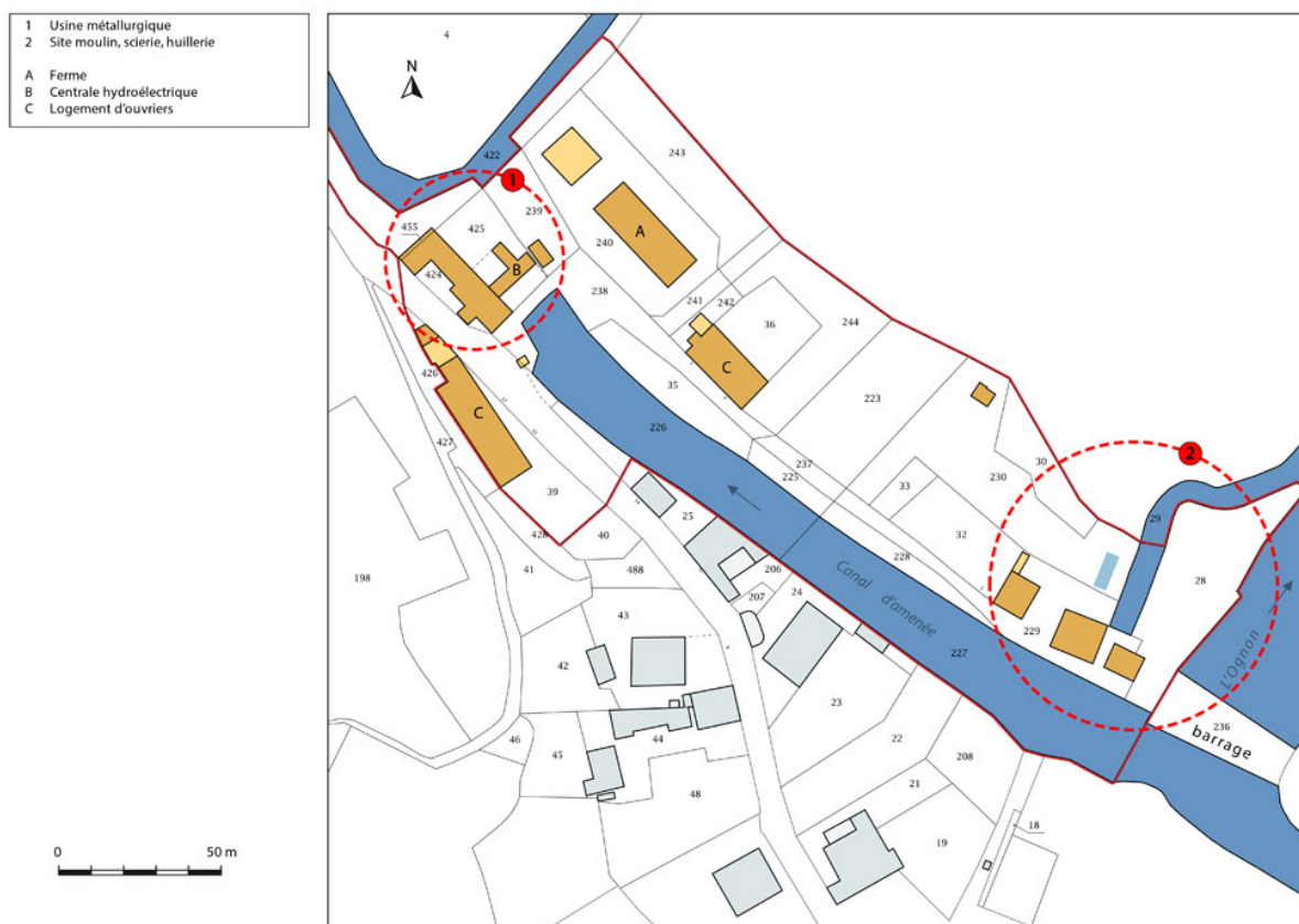
Plan-masse et de situation. Extrait du plan cadastral, 2016, section D.
