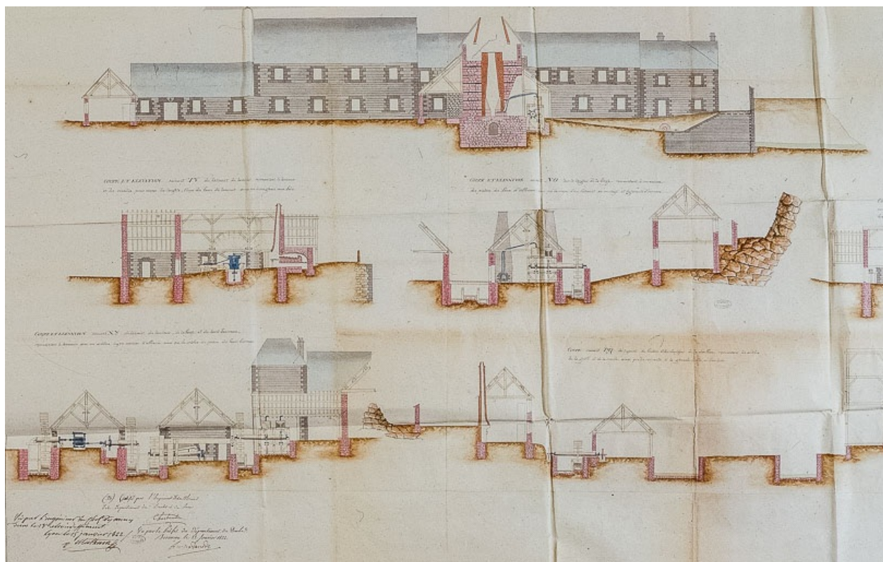
Coupe en long de l'atelier des laminoirs en 1821, par l'architecte Roland.
