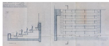
Coupe et plan des bancs de la tribune installés en gradins. Phot. Pierre-Marie Barbe- Richaud, Autr. Oskar Bitterli, Autr. Barnabé Augros IVR26_20227100256NUC2A
