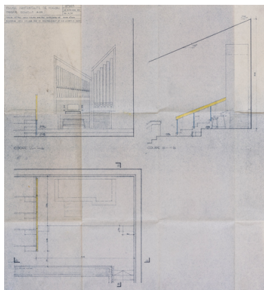
Plan et coupe de la tribune et élévation de l'orgue. Phot. Pierre-Marie Barbe- Richaud, Autr. Oskar Bitterli, Autr. Barnabé Augros IVR26_20227100253NUC2A
