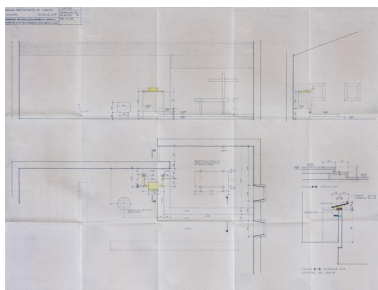
Plan, élévations et coupes de l'ambon, de la tribune, de la croix, de la table de communion, d'un banc et des fonts baptismaux. Phot. Pierre-Marie Barbe- Richaud, Autr. Oskar Bitterli, Autr. Barnabé Augros IVR26_20227100255NUC2A
