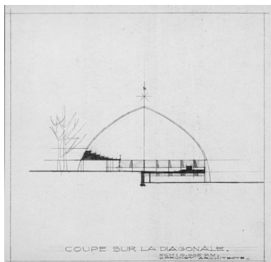
Coupe sur l'axe diagonal de l'église Sainte-Thérèse des Rosoirs. Autr. Pierre Prunet, Phot. Pierre-Marie Barbe-Richaud IVR26_20238900708NUC2A
