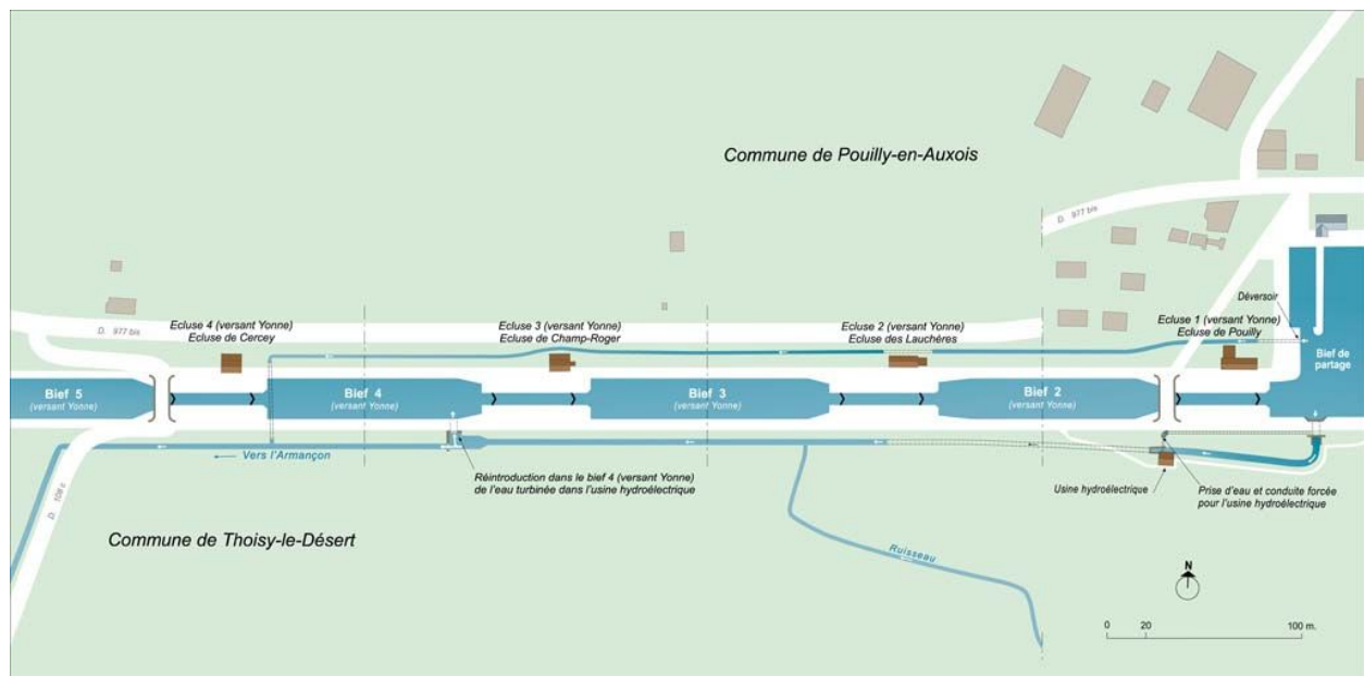
Plan schématique des biefs 01, 02 et 03 versant Yonne.
