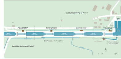
Plan schématique des biefs 01, 02 et 03 versant Yonne. Dess. Alain Morelière IVR26_20132100097NUDA
