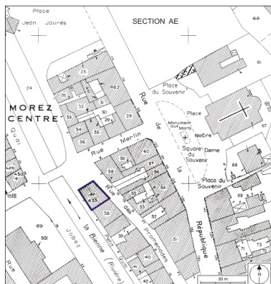
Plan-masse et de situation. Extrait du plan cadastral, 1980, section AI, échelle 1:1000. Dess. André Céréza IVR43_20093900279NUDA
