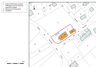
Plan-masse et de situation, section AD. Dess. Mathias Papigny IVR43_20142501904NUDA
