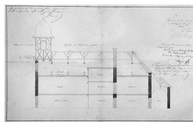
[Coupe de l'ancienne église montrant la charpente projetée], 1843. Phot. Jérôme Mongreville, Autr. Vital Ponard IVR43_19953900058X
