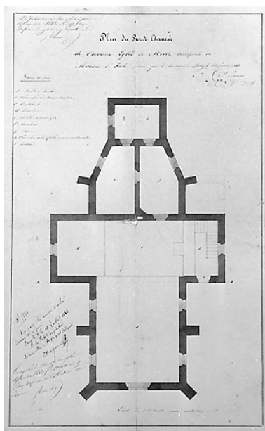
Plan du rez-de-chaussée de l'ancienne église de Morez transformée en maison d'école, 1843. Phot. Jérôme Mongreville, Autr. Vital Ponard IVR43_19953900057X
