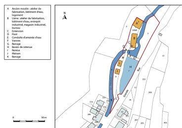
Plan-masse et de situation. Extrait du plan cadastral, 2017, section AC, 1/1 000. Dess. Mathias Papigny IVR43_20172501257NUDA
