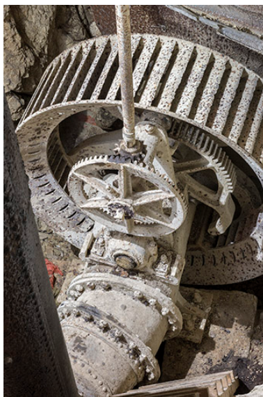
Usine : turbine Laurioz, au 2e étage de soubassement (chambre d'eau). Actionné depuis le rez- de-chaussée, l'arbre vertical commande l'admission d'eau. Phot. Sonia Dourlot IVR43_20172500031NUC4A
