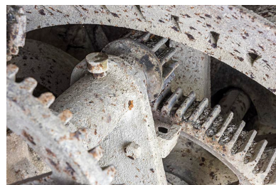
Usine : pignon entraînant le secteur commandant l'admission d'eau dans la turbine. Phot. Sonia Dourlot IVR43_20172500033NUC4A
