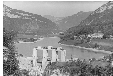
Barrage d'Etables et bassin de retenue. Phot. Jérôme Mongreville, Phot. Jules Manias IVR43_19963900177XI
