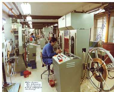
Atelier Presses des Ets Parrenin à Villers-le-Lac, décennie 1980. IVR43_20182500817NUC4A
