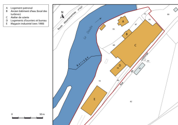
Plan-masse et de situation. Extrait du plan cadastral, 2015, section AB. Dess. Mathias Papigny IVR43_20162500941NUDA
