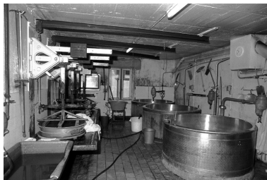
Intérieur de l'atelier de fabrication. Phot. Laurent Poupard IVR43_19923901297Z
