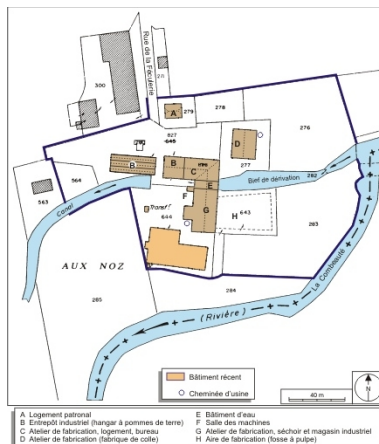
Plan-masse et de situation. Extrait du plan cadastral, 2008, section C, 1:1250 réduit à 1:1500. Source : Direction générale des Finances Publiques - Cadastre ; mise à jour : 2008. Dess. André Céréza IVR43_20087000212NUDA
