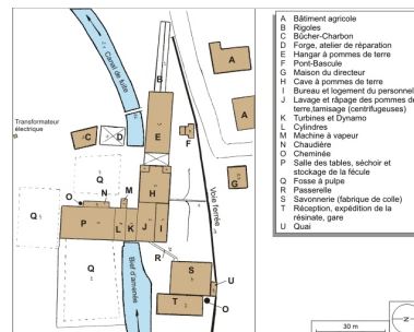
Plan-masse de la féculerie au début du 20e siècle. Dess. André Céréza IVR43_20087000213NUDA
