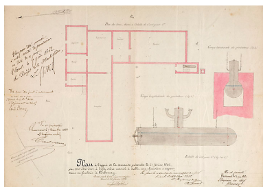
[Plan à l'appui de la demande présentée le 21 février 1862 par M. Poirson à l'effet d'être autorisé à établir une chaudière à vapeur dans sa féculerie à Corbenay]. Phot. Jérôme Mongreville IVR43_20077000042NUDA
