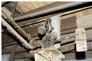
Régulateur à boules du système de transmission de la de la turbine. Phot. Jérôme Mongreville IVR43_20067000658NUCA
