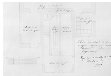
Plan du local de la chaudière à vapeur projetée par M. Erhard à Rougemont pour mouvoir un tissage mécanique. Phot. Jérôme Mongreville IVR43_20019000255X
