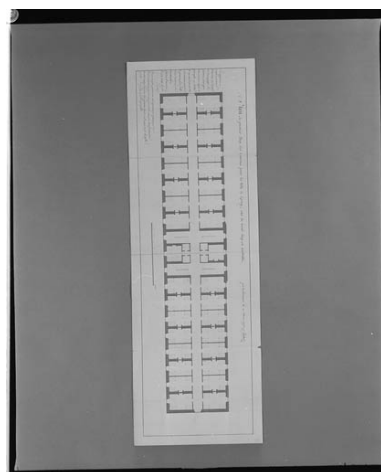
Plan du premier étage du bâtiment principal. Dessin, 1773. Phot. Yves Sancey, Autr. Louis (architecte) Aubert IVR43_19947000103X
