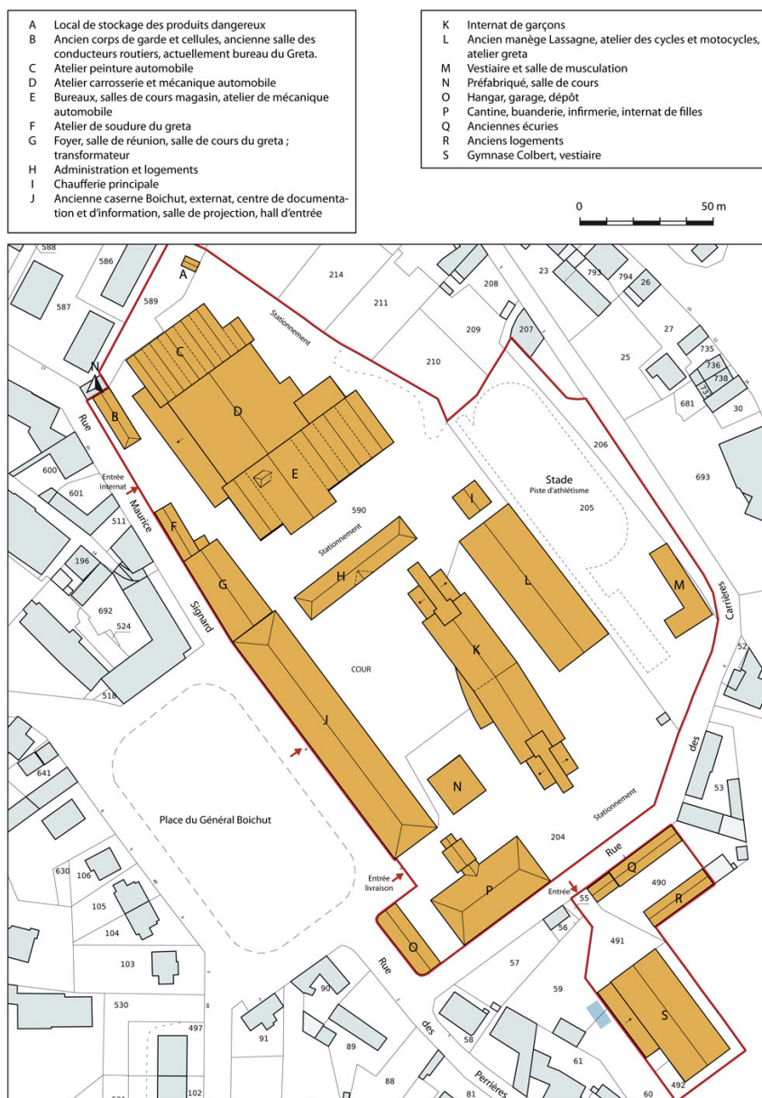
Plan-masse et de situation. Extrait du plan cadastral numérisé, section AB, échelle 1:1000.
