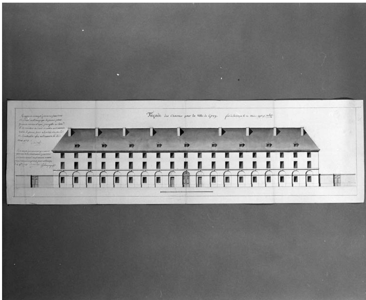
Elévation de la façade extérieure du bâtiment principal. Dessin, 1773.
