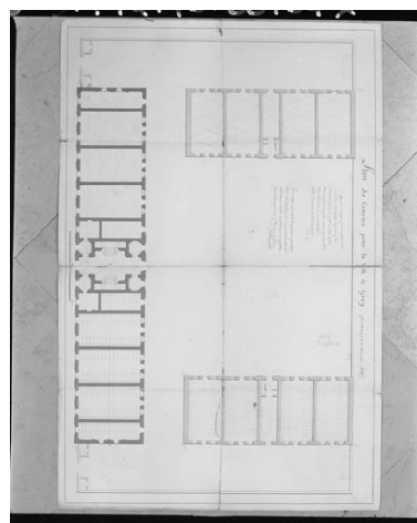
Plan du rez de chaussée. Dessin, 1773. Phot. Yves Sancey, Autr. Louis (architecte) Aubert IVR43_19947000104X
