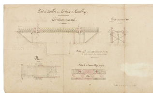
Ecluse d'Heuilley. Rétablissement du pont à treillis. Plans et détails. [Plan, coupe et élévation] 1871. Phot. Thierry Kuntz IVR26_20172100150NUC4A
