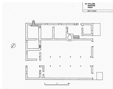
Plan au sol. Phot. Dominique et Sancey Dominguez IVR43_19792500016V
