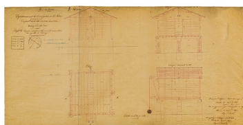
Projet de hangar insubmersible pour la conservation des aiguilles de barrage. [Plan, coupe et élévation]. 26 septembre 1847.
