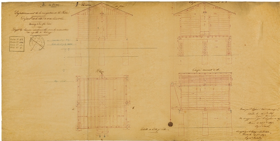
Projet de hangar insubmersible pour la conservation des aiguilles de barrage. [Plan, coupe et élévation]. 26 septembre 1847.
