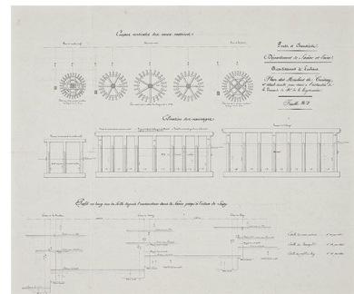
"Plan des moulins de Cuisery et détails divers pour servir à l'instruction de la demande de M. de la Teyssonnière, feuille n° 3 coupes verticales des roues motrices, élévation des vannes, profil en long depuis l'embouchure dans la Saône jusqu'à l'écluse de Loisy". Sans doute vers 1842. (Dessin, Archives VNF-direction territoriale Centre-Bourgogne ; subdivision de Montceau-les-Mines)
