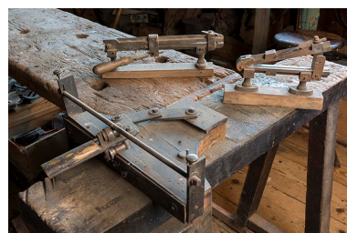
Atelier : machine à redresser les barres et autres machines. Phot. Sonia Dourlot IVR43_20172500788NUC4A
