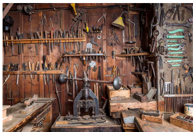
Atelier : outils et presse à balancier. Phot. Sonia Dourlot IVR43_20172500785NUC4A
