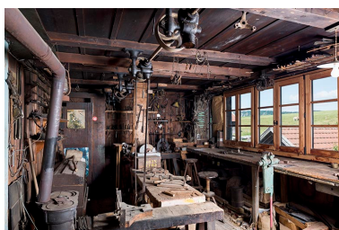
Atelier à l'étage : vue d'ensemble. Phot. Sonia Dourlot IVR43_20172500783NUC4A
