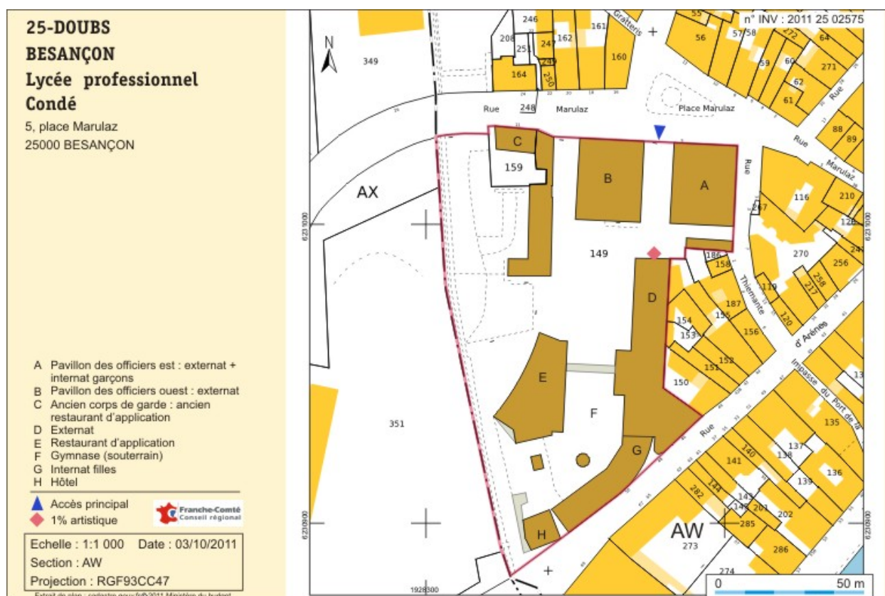
Plan-masse et de situation. Extrait du plan cadastral numérisé, section AX, échelle 1:1000
