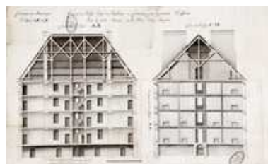
Coupes du corps de casernes à construire. Dessin aquarellé : 40,3 x 65,4 cm, 1738. Phot. Jérôme Mongreville IVR43_20112502616NUC4A
