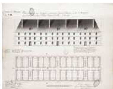
Plan et élévation du corps de casernes à construire. Dessin aquarellé : 51,3 x 67,6 cm, 1738. Phot. Jérôme Mongreville IVR43_20112502611NUC4A
