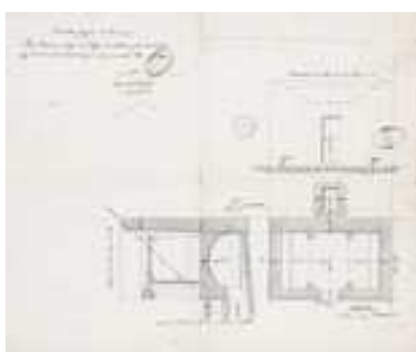
Plan, élévation et coupe des latrines pour les soldats. Dessin aquarellé, 1738. Phot. Jérôme Mongreville IVR43_20112502612NUC4A
