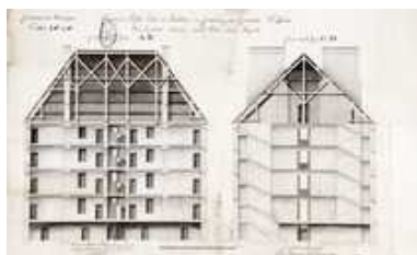
Coupes du corps de casernes à construire. Dessin aquarellé : 40,3 x 65,4 cm, 1738. Phot. Jérôme Mongreville
