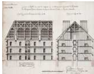
Coupes de la caserne à construire. Dessin aquarellé : 43,8 x 55,7 cm, 1738. Phot. Jérôme Mongreville IVR43_20112502610NUC4A
