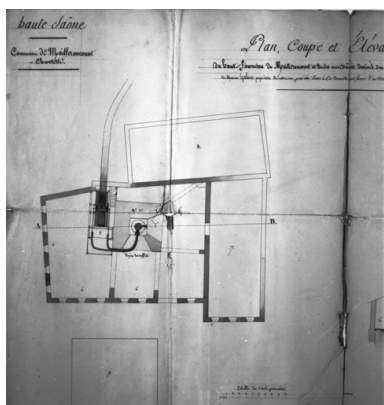
Plan, coupe et élévation du haut fourneau de Mailleroncourt et de ses accessoires [...] Phot. Jérôme Mongreville IVR43_19877000043X
