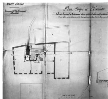
Plan, coupe et élévation du haut fourneau de Mailleroncourt et de ses accessoires [détail du haut fourneau]. Phot. Jérôme Mongreville IVR43_19877000045X
