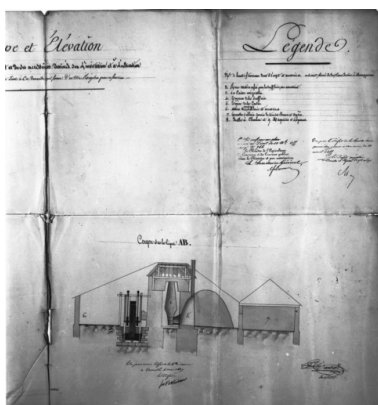
Plan, coupe et élévation du haut fourneau de Mailleroncourt et de ses accessoires [coupe transversale]. Phot. Jérôme Mongreville IVR43_19877000044X
