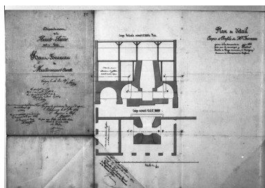
Haut fourneau de Mailleroncourt-Charette. Plan de détail, coupes et profils du haut fourneau. Phot. Jérôme Mongreville IVR43_19877000046X
