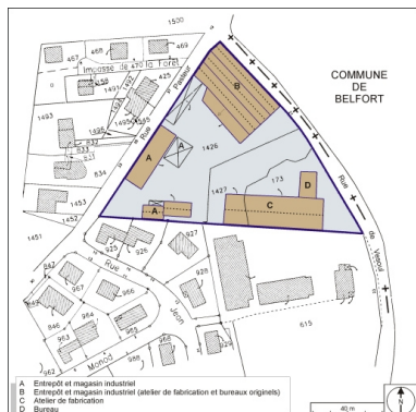
Plan-masse et de situation. Extrait du plan cadastral, 2001, section A, 1:1250. Dess. André Céréza IVR43_20039000022NUDA
