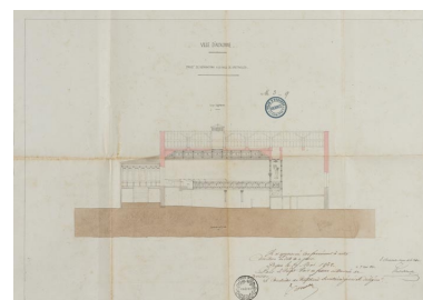
Ville d'Auxonne. Projets de réparations à la salle de spectacle. [Coupe longitudinale]. 3 mai 1842. Phot. Pierre-Marie Barbe- Richaud, Autr. Claude Phal-Blando IVR26_20212100053NUC4A
