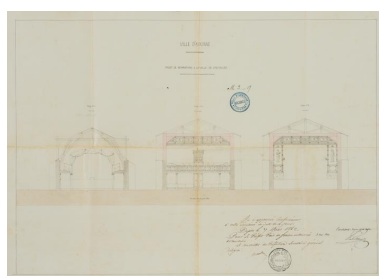
Ville d'Auxonne. Projets de réparations à la salle de spectacle. [Coupe transversale]. 3 mai 1842. Phot. Pierre-Marie Barbe- Richaud, Autr. Claude Phal-Blando IVR26_20212100055NUC2A
