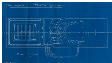
Ville d'Auxonne. Théâtre municipal. Plan étage. Phot. Pierre-Marie Barbe-Richaud, Autr. auteur inconnu IVR26_20212100048NUC2A
