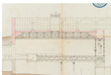
Ville d'Auxonne. Projets de réparations à la salle de spectacle. [Détail de la coupe longitudinale]. 3 mai 1842. Phot. Pierre-Marie Barbe- Richaud, Autr. Claude Phal-Blando IVR26_20212100054NUC4A
