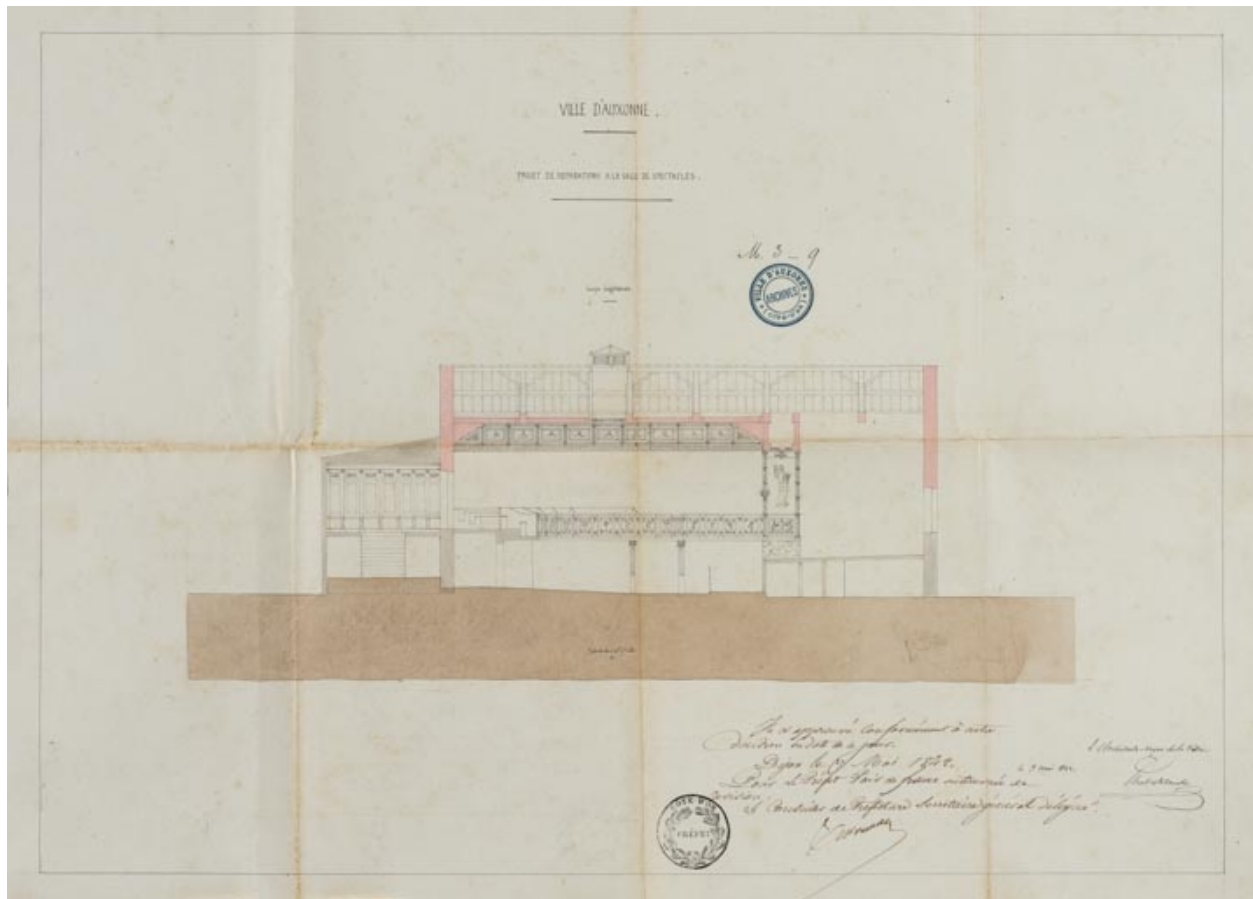
Ville d'Auxonne. Projets de réparations à la salle de spectacle. [Coupe longitudinale]. 3 mai 1842.
