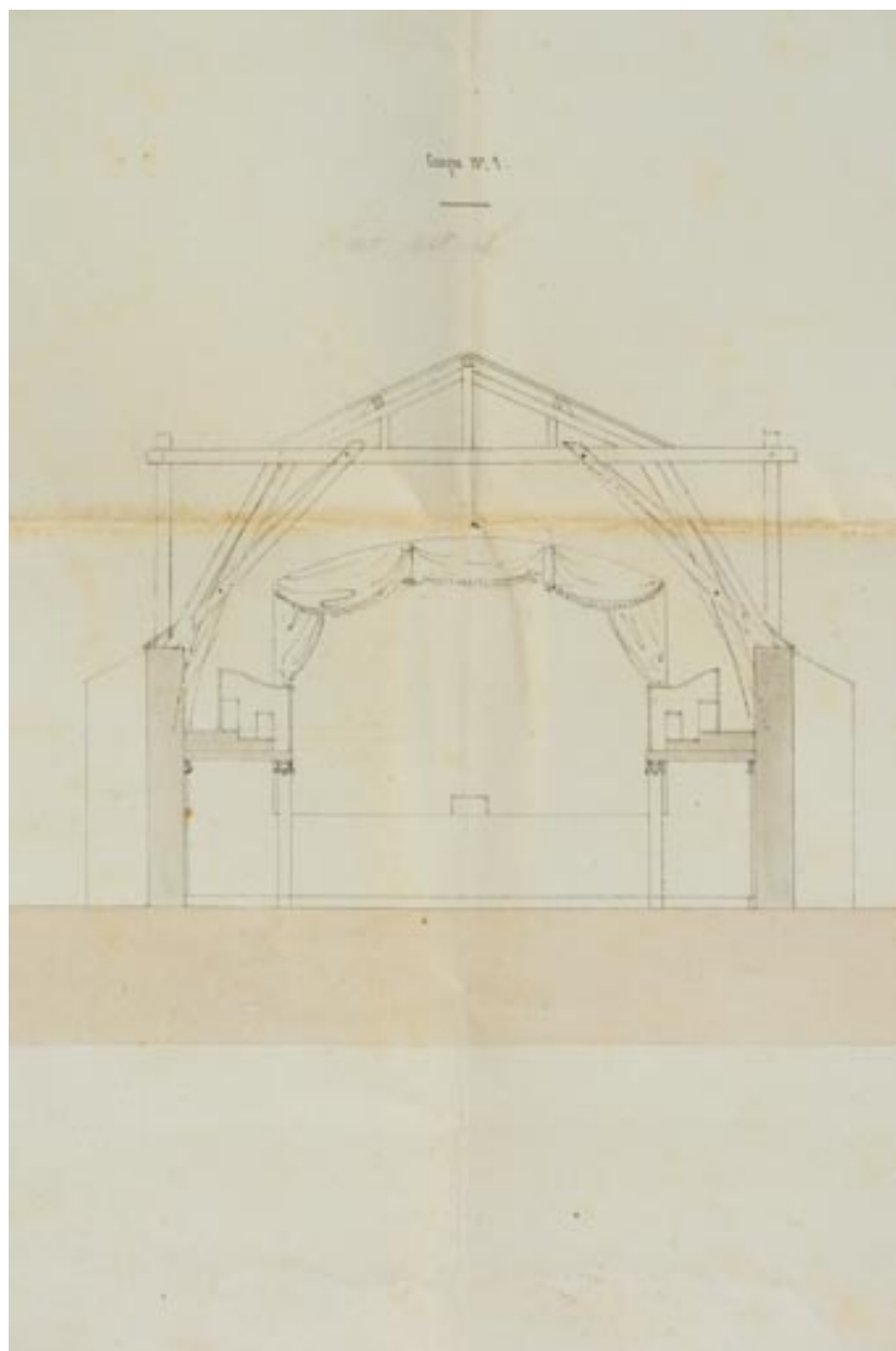
Ville d'Auxonne. Projets de réparations à la salle de spectacle. [Détail de la coupe transversale : avant transformation]. 3 mai 1842.
