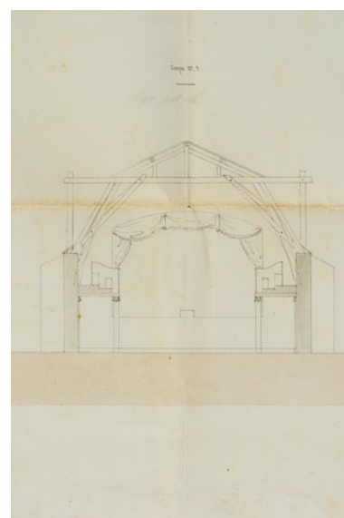
Ville d'Auxonne. Projets de réparations à la salle de spectacle. [Détail de la coupe transversale : avant transformation]. 3 mai 1842. Phot. Pierre-Marie Barbe- Richaud, Autr. Claude Phal-Blando IVR26_20212100056NUC4A
