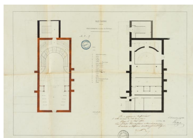
Ville d'Auxonne. Projets de réparations à la salle de spectacle. [Plan]. 3 mai 1842. Phot. Pierre-Marie Barbe- Richaud, Autr. Claude Phal-Blando IVR26_20212100052NUC4A
