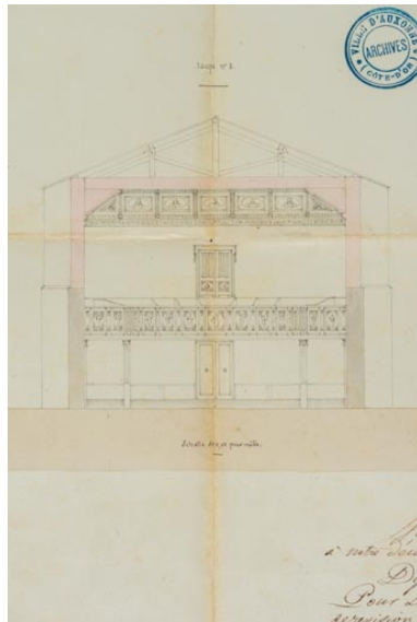
Ville d'Auxonne. Projets de réparations à la salle de spectacle. [Détail de la coupe transversale : côté entrée]. 3 mai 1842. Phot. Pierre-Marie Barbe-Richaud, Autr. Claude Phal-Blando IVR26_20212100057NUC4A
