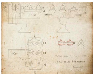
Machine à pivoter. Grandeur exécutive, septembre 1916.
