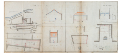
Plan des lavoirs du Théâtre, de la Fourmandaise et de Galvoz, 1879. Phot. Jérôme Mongreville IVR43_20233900914NUC4A
