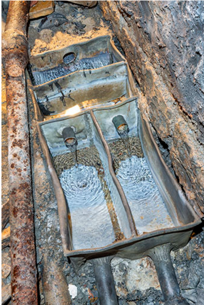
Bassins de division en plomb.
