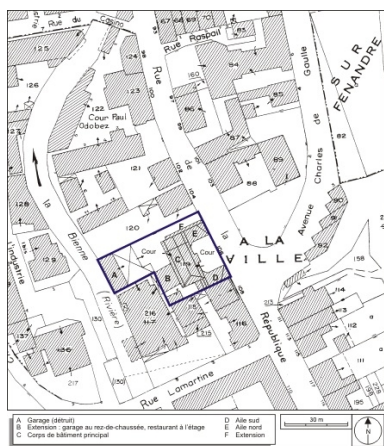
Plan-masse et de situation. Extrait du plan cadastral, 1980, section AE, échelle 1:1000. Dess. André Céréza IVR43_20093900240NUDA
