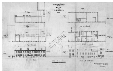
Montbéliard. Plan de l'hôpital [à gauche corps de bâtiment sur la rue du Château, à droite corps de bâtiment sur la Schiffe], 1898. Phot. Jérôme Mongreville, Autr. Parrot IVR43_19872500221X
