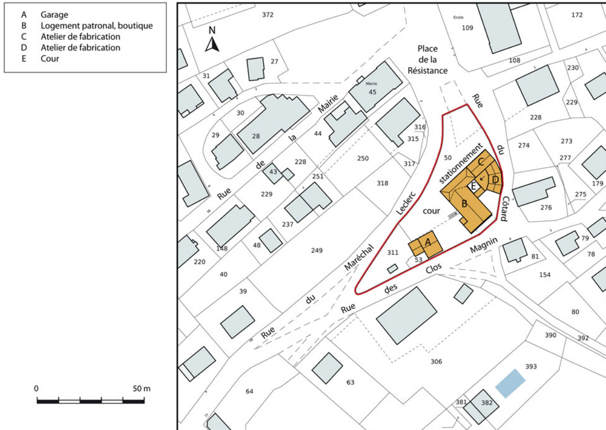
Plan-masse et de situation. Extrait du plan cadastral, 2012, section AE.
