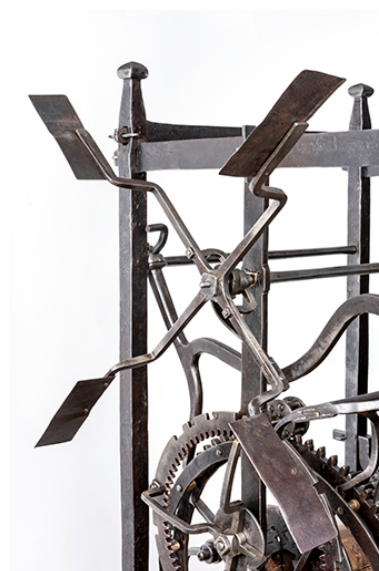
Détail de l'horloge publique : le volant régulateur de sonnerie.
