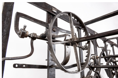
Détail du mécanisme d'horloge : l'échappement.
