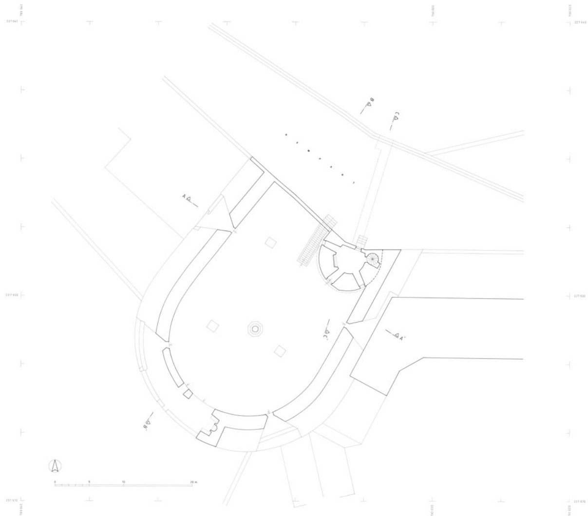
Plan sur terrasse du boulevard et du niveau supérieur de la tour des Cordeliers.
