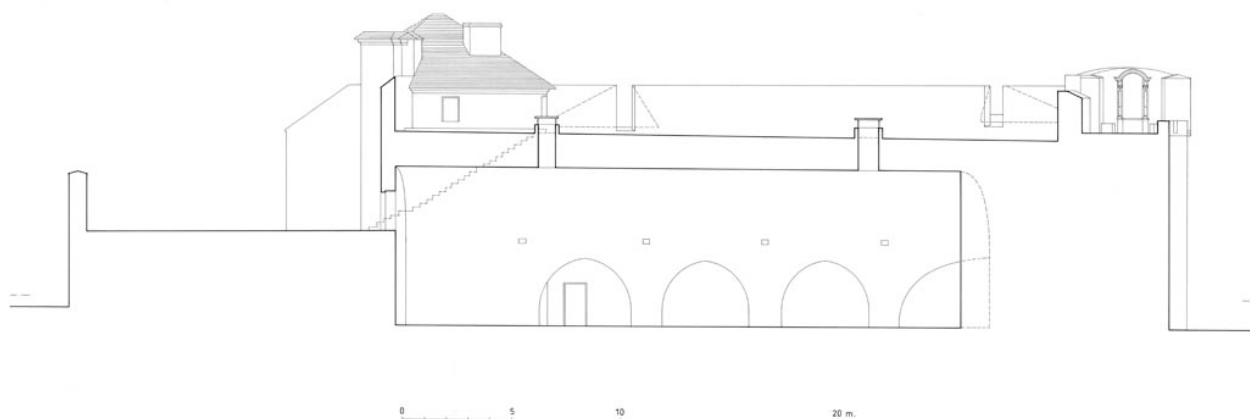
Grosse tour boulevard, improprement appelé bastion de l'Hôtel-Dieu : coupe transversale.
