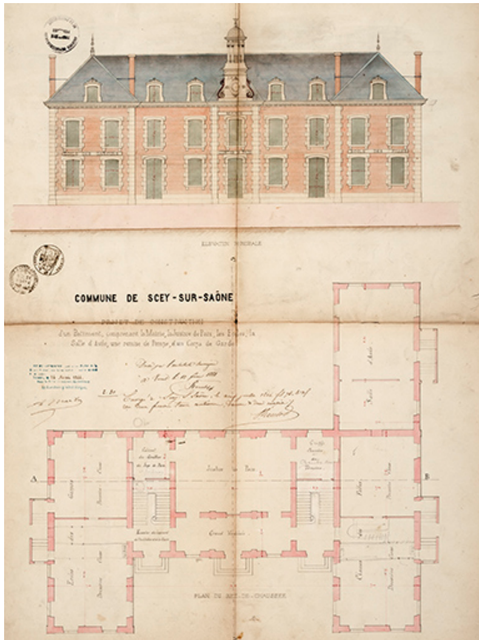
Renahy. Élévation et plan du rez-de-chaussée. 1866.
