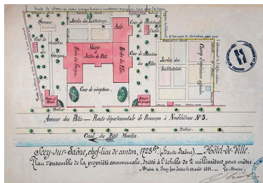
Hôtel de Ville. Plan d'ensemble de la propriété communale. 1881. Repro. Jérôme Mongreville, Autr. auteur inconnu IVR43_20197000036NUC4A
