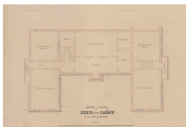
Hôtel de Ville de Scey-sur-Saône. Plan du rez-de-chaussée. [1888]. Autr. auteur inconnu IVR43_20197000150NUCA
