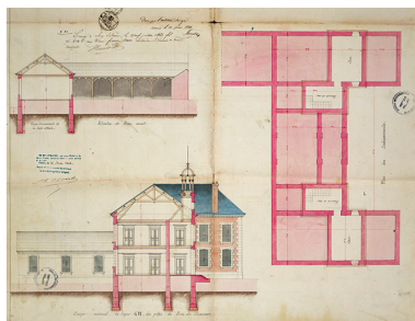
Renahy. Projet de construction d'une maison commune, coupes et plan des soubassements. 1866. Repro. Jérôme Mongreville, Autr. Adrien Renahy IVR43_20197000012NUC4A
