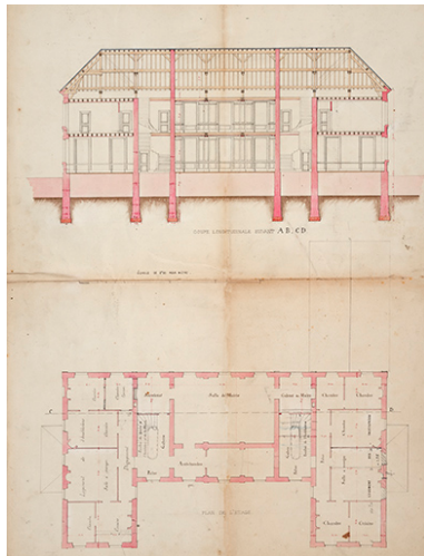
Renahy. Coupe longitudinale et plan de l'étage. 1866. Repro. Jérôme Mongreville, Autr. Adrien Renahy IVR43_2019700007NUC4A
