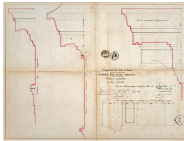
Renahy. Profil de corniche au demi d'exécution. 1866. Repro. Jérôme Mongreville, Autr. Adrien Renahy IVR43_20197000014NUC4A
