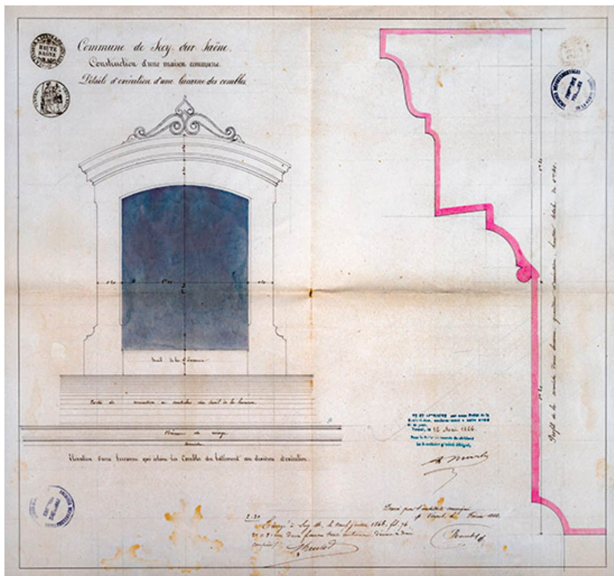
Renahy. Lucarne des combles. 1866.
