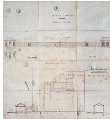
Renahy. Construction d'un hôtel de Ville. 1866. Repro. Jérôme Mongreville, Autr. Adrien Renahy IVR43_20197000042NUC4A
