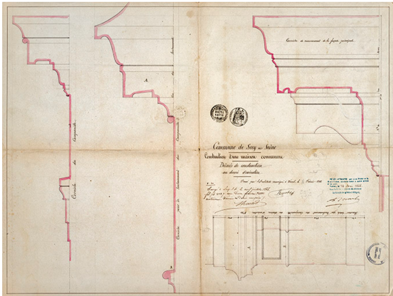
Renahy. Profil de corniche au demi d'exécution. 1866.
