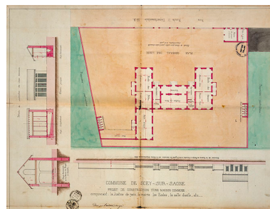
Renahy. Plan général, coupe et plan des lieux d'aisances et de la remise des pompes à incendie. 1866. Repro. Jérôme Mongreville, Autr. Adrien Renahy IVR43_20197000013NUC4A
