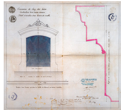
Renahy. Lucarne des combles. 1866. Repro. Jérôme Mongreville, Autr. Adrien Renahy IVR43_20197000018NUC4A
