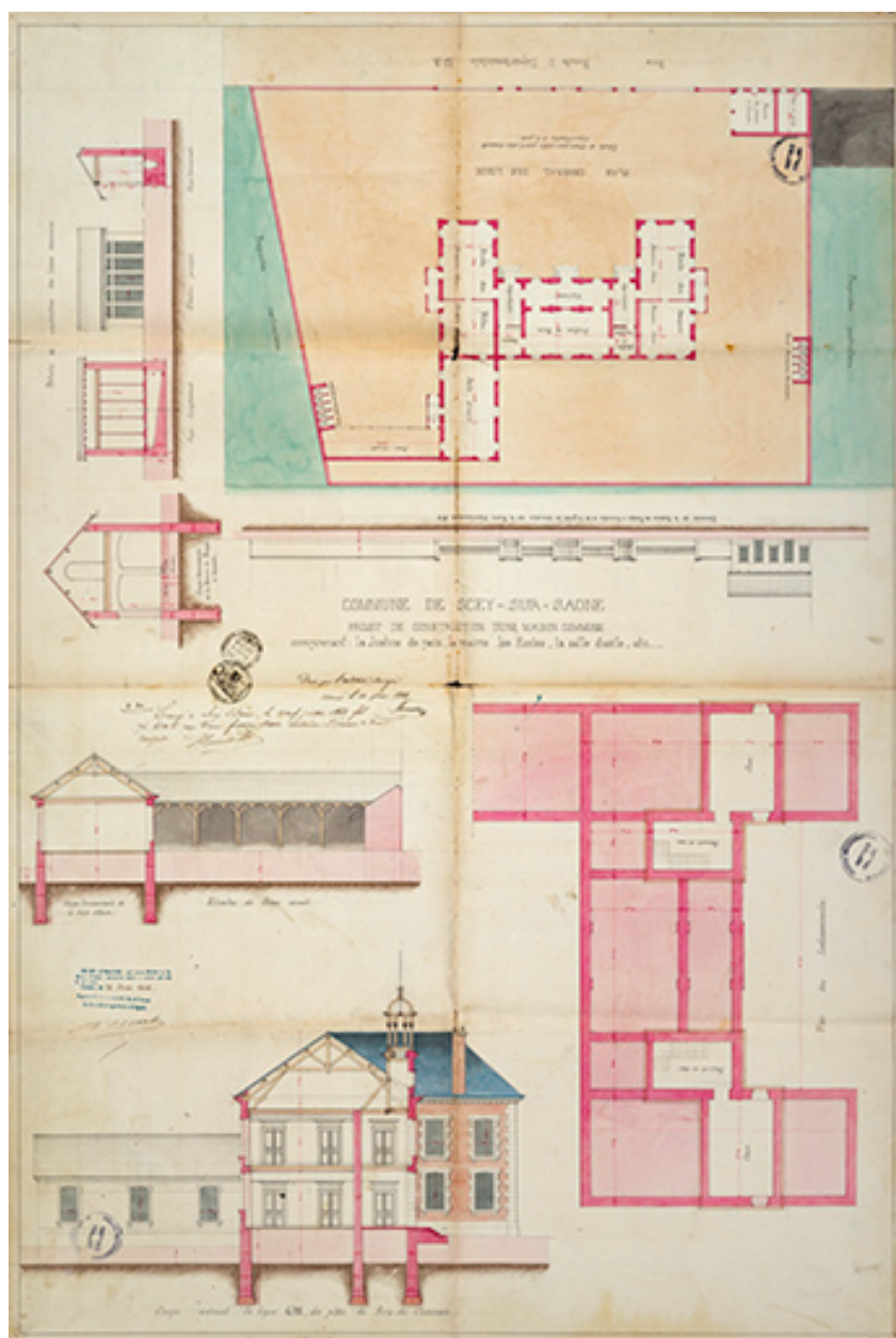
Renahy. Projet de construction d'une maison commune. 1866.
