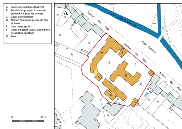
Plan-masse et de situation. Extrait du plan cadastral, 2019. Dess. Bertrand Turina IVR43_20197000223NUDA
