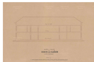
Hôtel de Ville de Scey-sur- Saône. Coupe verticale. [1888]. Autr. auteur inconnu IVR43_20197000152NUCA
