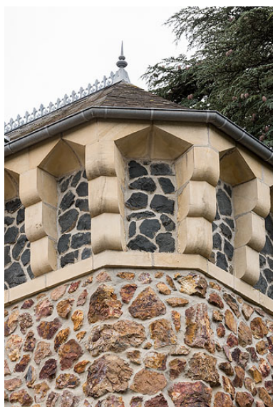
Détail de la tour de plan rectangulaire. Phot. Pierre-Marie Barbe-Richaud IVR26_20205800265NUC4A
