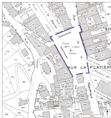
Plan de situation. Extrait du plan cadastral, 1980, section AI, échelle 1:1000. Dess. André Céréza
