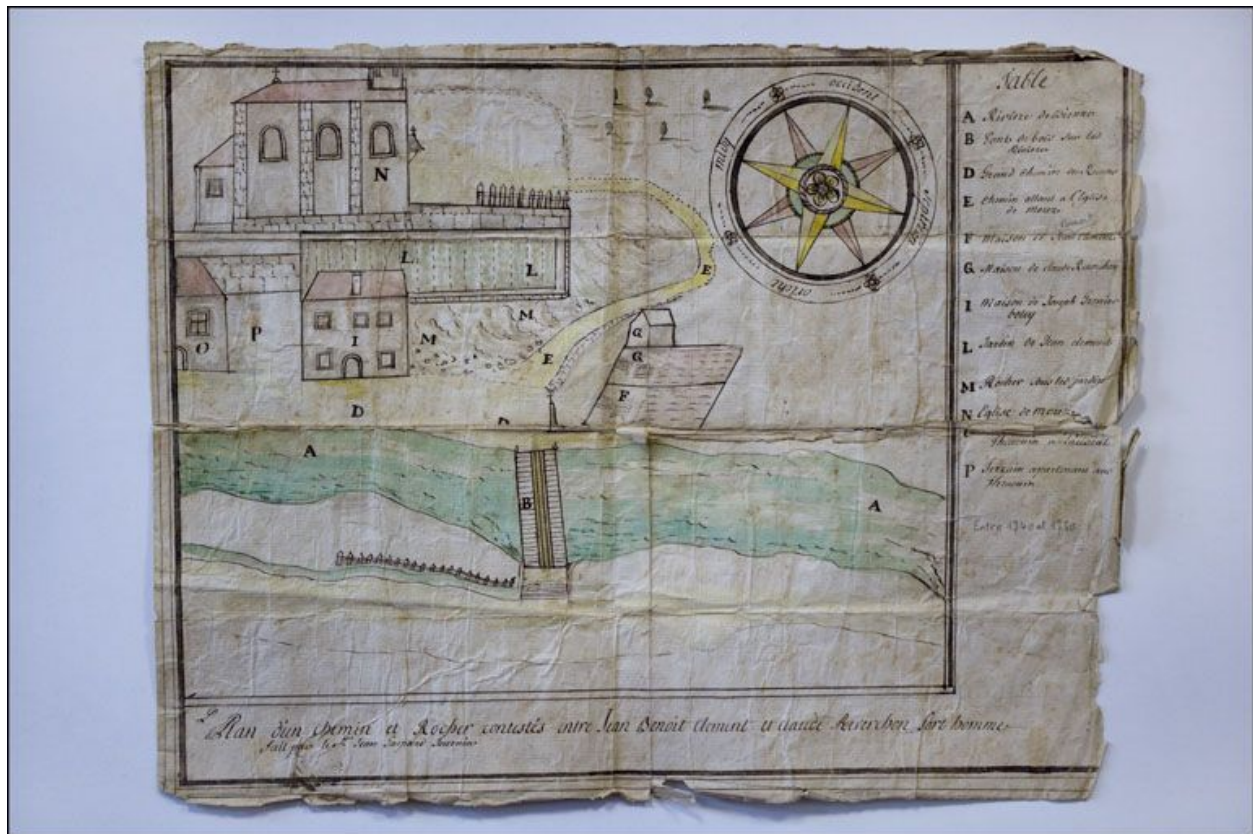
Plan d'un chemin et rocher contestés entre Jean Benoit Clément et Claude Reverchon fort homme, entre 1740 et 1750. Dessin (plume, lavis), s.d. [entre 1740 et 1750], sans échelle.
