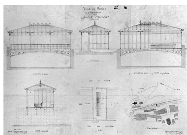
Construction d'un lavoir couvert [projet non réalisé de lavoir enjambant la Bienne], 1877. Phot. Jérôme Mongreville, Phot. Paillot IVR43_19953900063X
