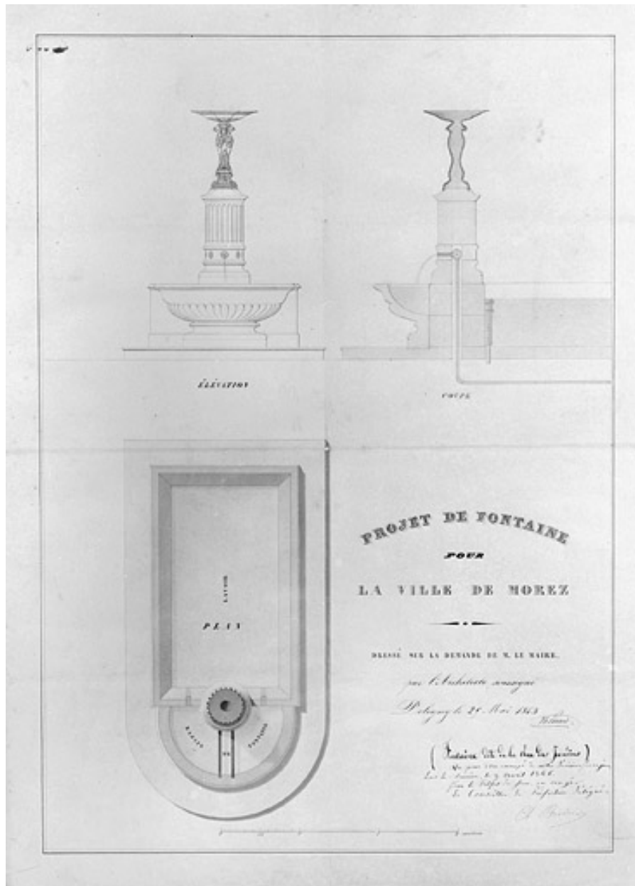
Projet de fontaine pour la ville de Morez (Fontaine dite de la Rue des Jardins) [projet non réalisé], 1843.
