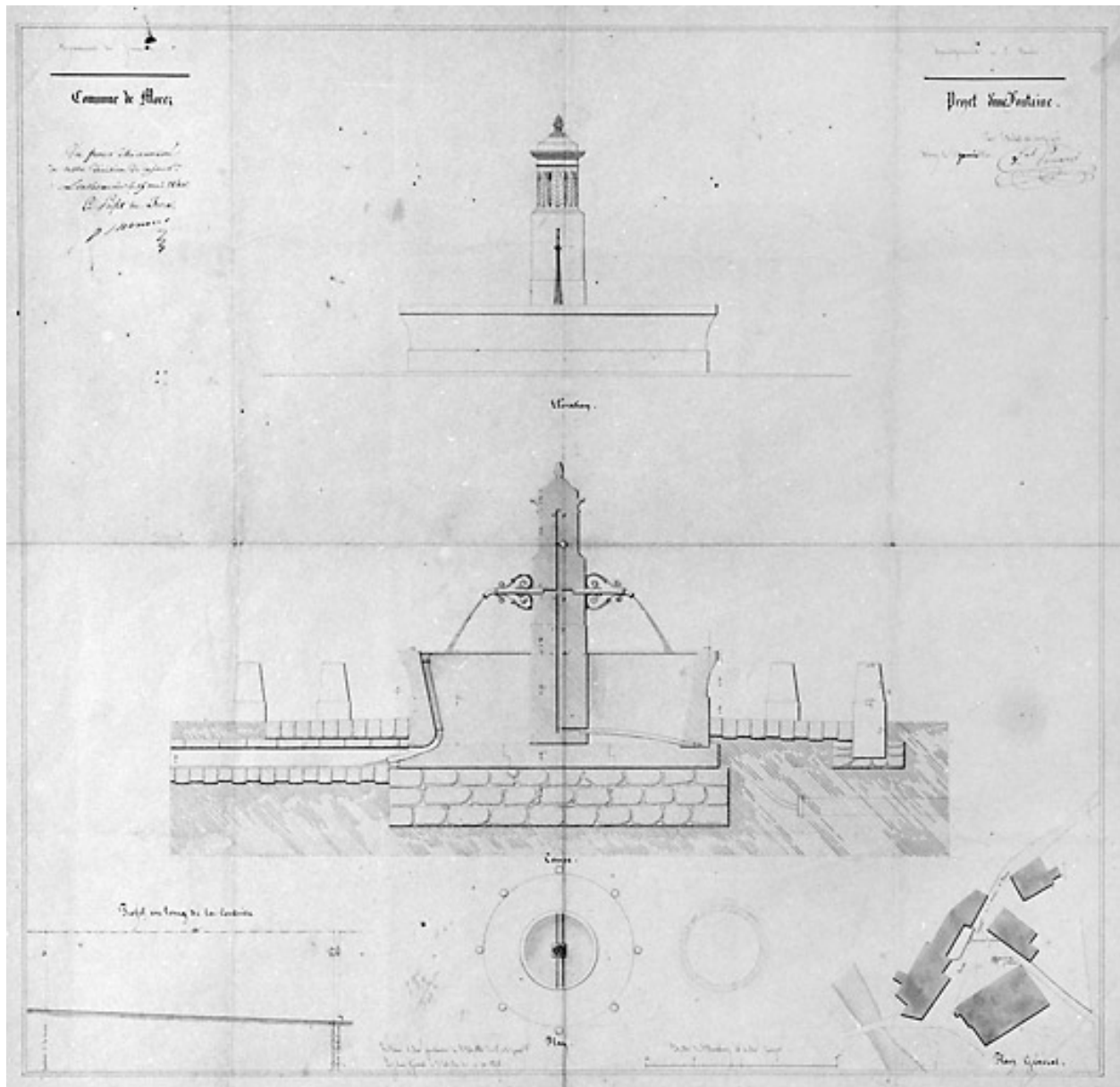
Commune de Morez. Projet d'une fontaine [place de la Samaritaine, actuellement Jules Girod], 1840.
