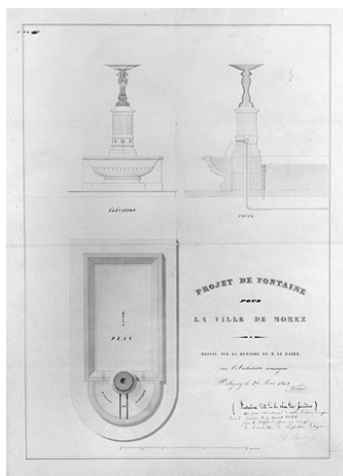
Projet de fontaine pour la ville de Morez (Fontaine dite de la Rue des Jardins) [projet non réalisé], 1843. Phot. Jérôme Mongreville, Phot. Narcisse Perrard IVR43_19953900027V
