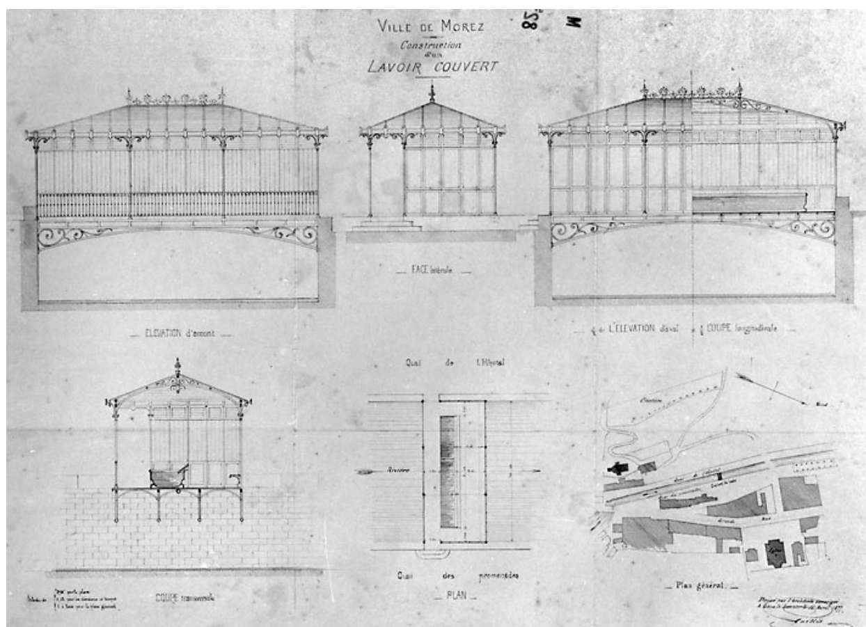
Construction d'un lavoir couvert [projet non réalisé de lavoir enjambant la Bienne], 1877.
