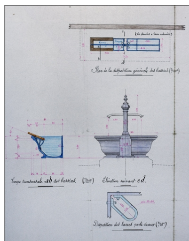
Etablissement de bassins en fonte au lavoir public dit de l'Hôpital. Dessins, 1912. Phot. Yves Sancey, Phot. Lacroix IVR43_20103900055NUC2A
