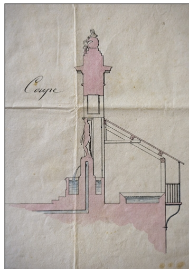
Commune de Morez. Projet d'une fontaine [place de la Samaritaine, actuellement Jules Girod], 1840. Phot. Jérôme Mongreville, Autr. Vital (architecte) NEPASUTILISER IVR43_19953900065X
