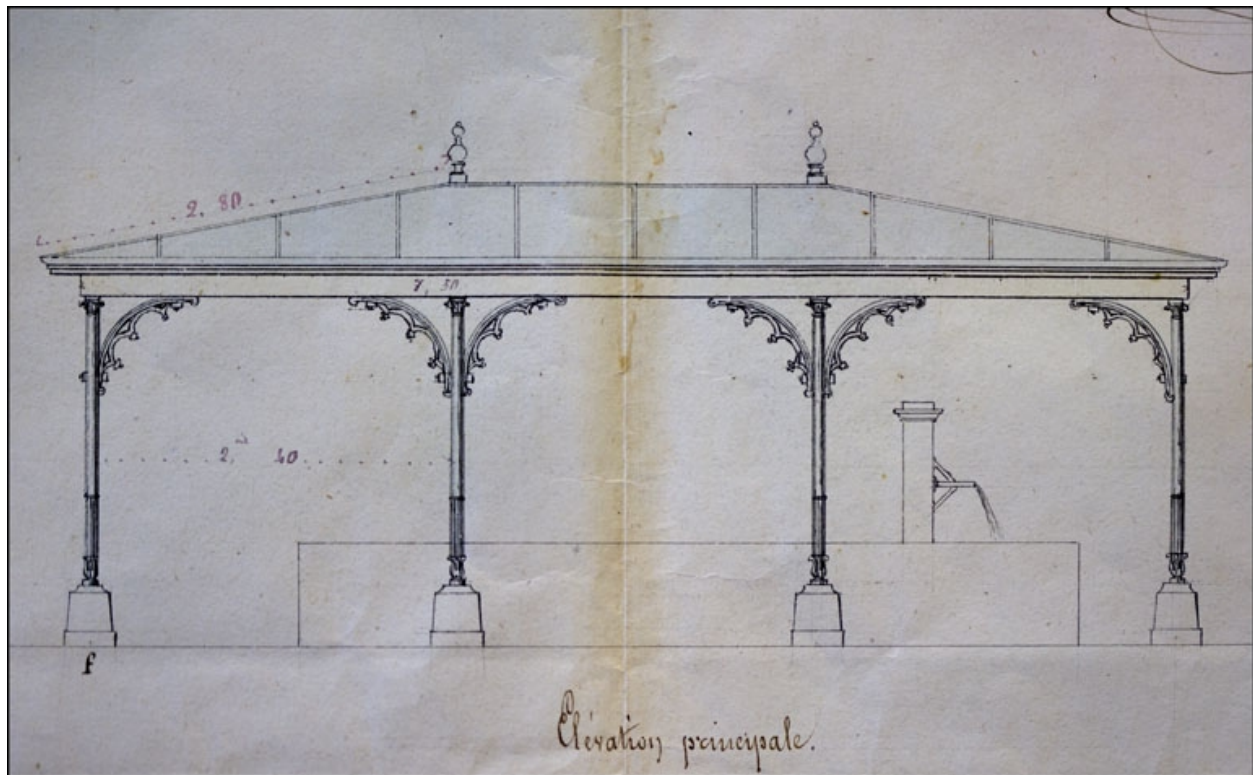
Projet d'une toiture pour un lavoir public (Quai de l'ancienne place). [Détail :] Elévation principale, 1850.
