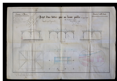
Projet d'une toiture pour un lavoir public (Quai de l'ancienne place), 1850. Phot. Yves Sancey, Phot. Vital Ponard IVR43_20103900067NUC2A
