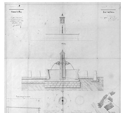
Commune de Morez. Projet d'une fontaine [place de la Samaritaine, actuellement Jules Girod], 1840. Phot. Jérôme Mongreville, Autr. Vital (architecte) NEPASUTILISER IVR43_19953900065X
