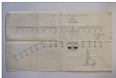
Fontaine Lavoir et Echopes à construire à Morez, 1819. Phot. Yves Sancey, Phot. Denis-Philibert Lapret IVR43_20103900016NUC2A
