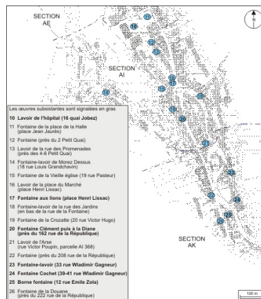
Plan de localisation : partie sud. Montage de feuilles cadastrales, 1980, sections AE, AI et AK, échelle 1:1000 réduite à 1:6000. Dess. André Céréza IVR43_20103900191NUDA
